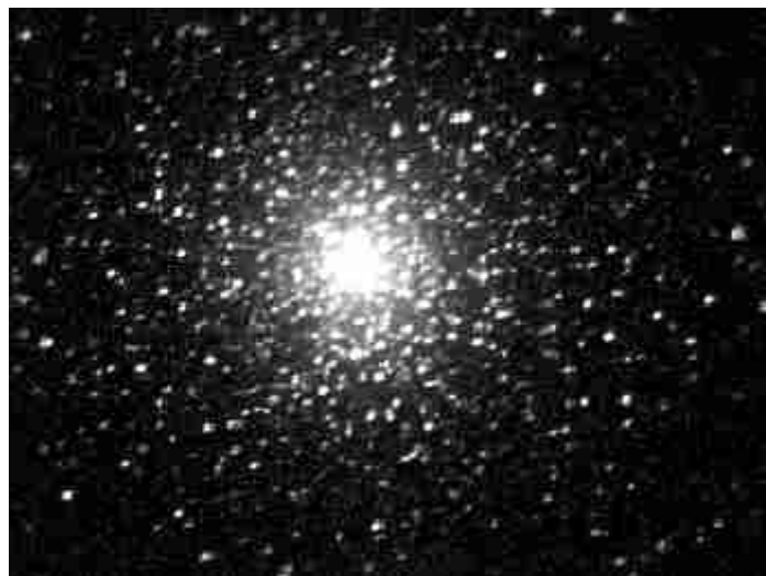
M15, cúmulo globular en Pegasus, situado a 34.000 años-luz. Por tratarse de un objeto difuso, se ve rápidamente afectado por la contaminación lumínica. Foto Pere Horts
